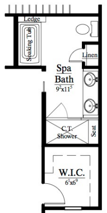
Optional Spa Bath 2
